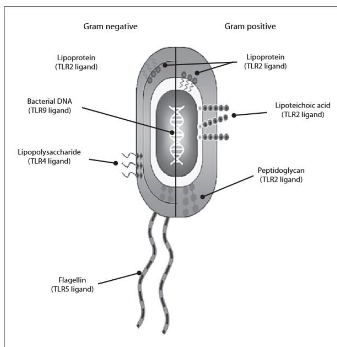
Рисунок 5 - Toll-подобные рецепторы взаимодействуют с соответствующими патоген-ассоциированными молекулярными структурами (PAMPs) бактерий [177]
