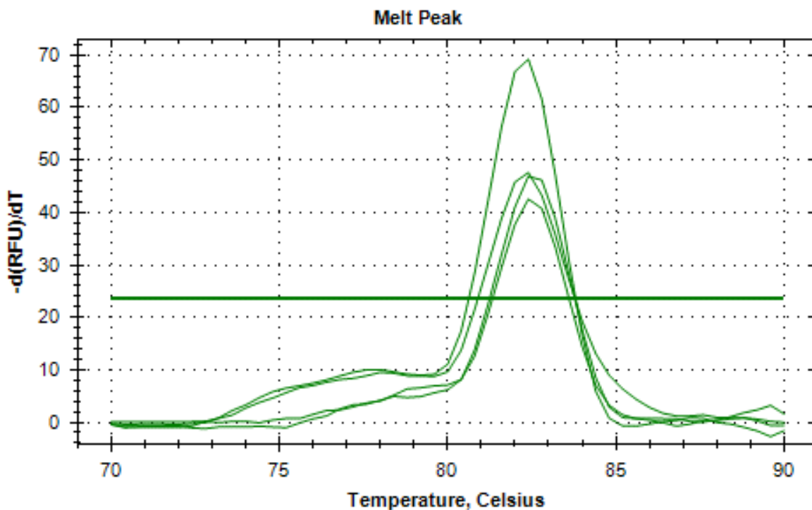
Рисунок 20 - Кривые плавления в тестируемых образцах в образцах E. coli тканями мезентериальных лимфатических узлов на этапе качественного определения наличия микроорганизмов в МЛЮ (Temperature, Celsius – температура в градусах Цельсия, d(RFU)/dT - отрицательная скорость изменения относительной единицы флуоресценции при изменении температуры)
