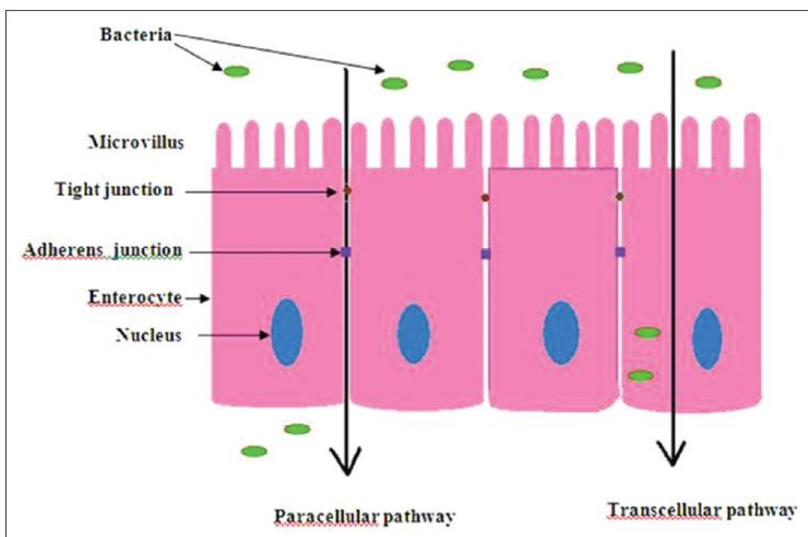
Рисунок 2 - Схематичное изображение прохождения бактерий через кишечный барьер трансклеточным (transcellular pathway) и параклеточным (paracellular pathway) путями. Bacteria – бактериальный агент, Microvillus – микроворсинки, Tight junction – плотные соединения, Adherens junction - соединение адгезивов, Enterocyte – энтероцит, Nucleus – ядро энтероцита [57]
