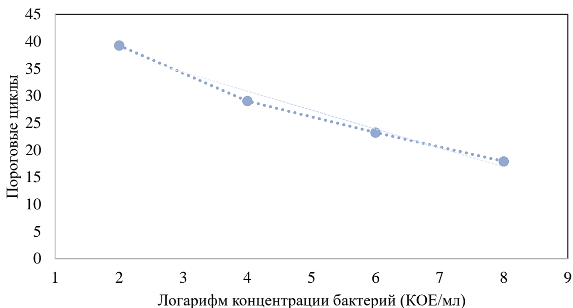
Рисунок 25 – Кривая стандартов ПЦР в группе E. coli с КОЕ/мл от 10^2 до 10^8 совместно с тканью мезентериальных лимфатических узлов ( y = – уравнение линейной регрессии согласно разработанной математической модели, R^2 - коэффициент детерминации)
