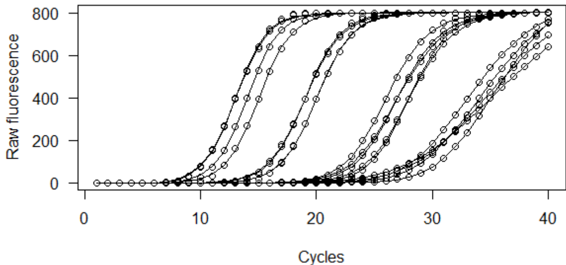
Рисунок 22 – Графики амплификации образцов E. coli с КОЕ/мл 10^2 , 10^4 , 10^6 , 10^8 в физиологическом растворе (Raw fluorescence - относительная единица флуоресценции, Cycles - циклы амплификации)
