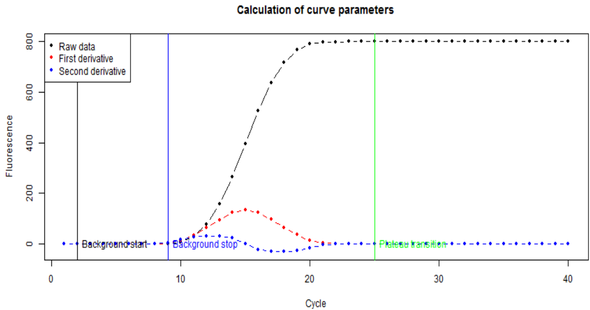
Рисунок 21 - График амплификации на основе сигмоидной модели с 4 параметрами и рассчитанные пороговые циклы на основе производной нелинейной модели, а также эффективность амплификации. (Первая производная – красная линия, вторая производная – синяя линия, график амплификации - черная линия)
