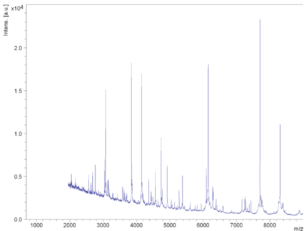
Рисунок 18 – Результаты MALDI-TOF MS, соответствующие детекции бактерий Klebsiella (Intens. – интенсивность пика, m/z – отношение массы к заряду)
