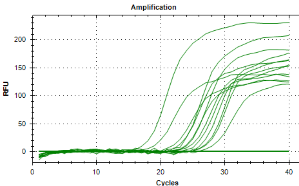
Рисунок 19 - Графики амплификации тестируемых образцов на этапе качественного определения наличия микроорганизмов в МЛУ (RFU - относительная единица флуоресценции, Cycles - циклы амплификации)
