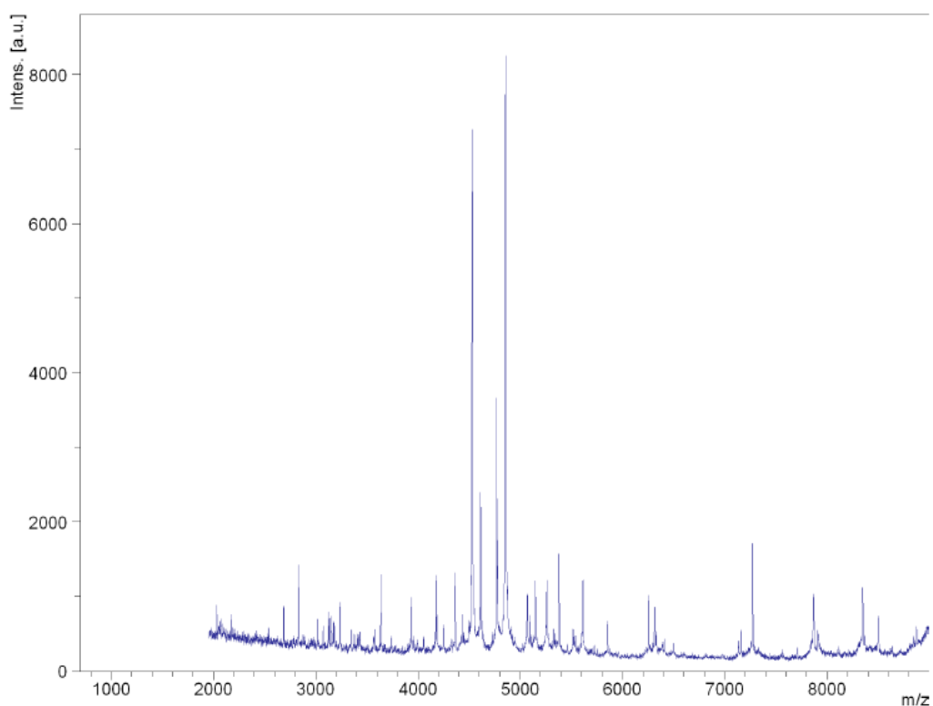
Рисунок 17 – Результаты MALDI-TOF MS, соответствующие детекции бактерий Escherichia coli (Intens. – интенсивность пика, m/z – отношение массы к заряду)
