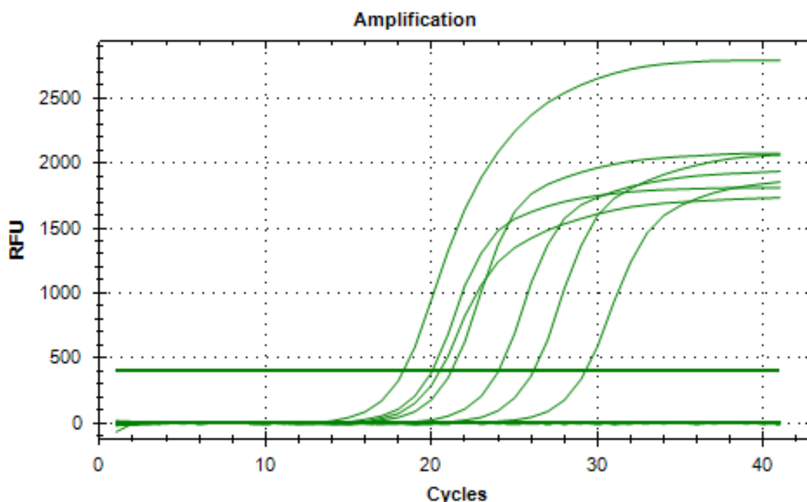
Рисунок 26 -Графики амплификации образцов МЛУ пациентов с КРР с положительным результатом ПЦР (RFU - относительная единица флуоресценции, Cycles - циклы амплификации)
