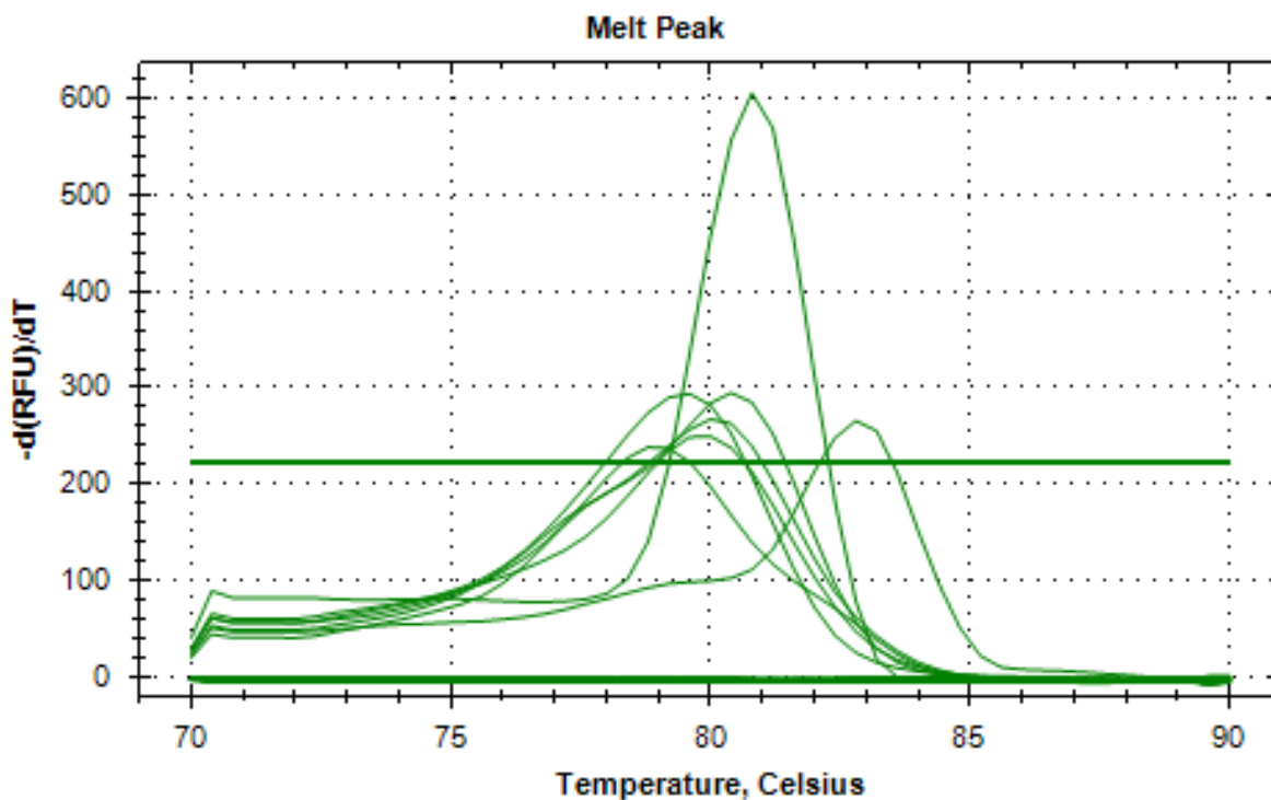
Рисунок 27 - Кривые плавления в образцах МЛУ пациентов с КРР с положительным результатом ПЦР (Temperature, Celsius – температура в градусах Цельсия, d(RFU)/dT - отрицательная скорость изменения относительной единицы флуоресценции при изменении температуры)
