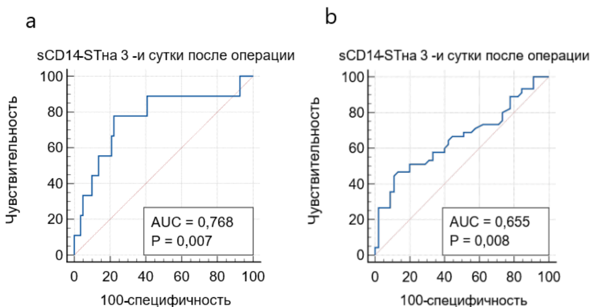
Рисунок 38 – ROC-кривые уровня sCD14-ST на 3-и сутки после оперативного вмешательства для прогнозирования летального исхода (а), стадии опухолевого процесса (b)
