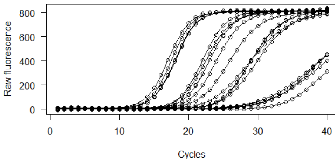
Рисунок 23 – Графики амплификации образцов E. coli с КОЕ/мл 10^2 , 10^4 , 10^6 , 10^8 с тканями мезентериальных лимфатических узлов (Raw fluorescence - относительная единица флуоресценции, Cycles - циклы амплификации)
